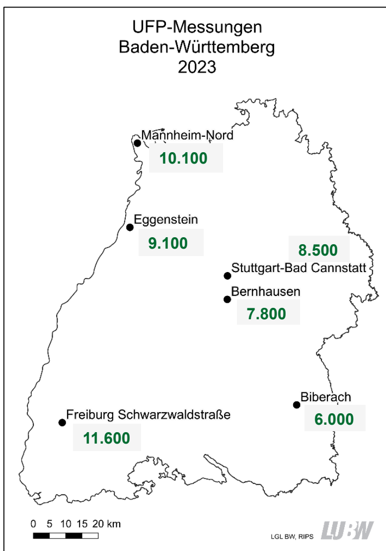
Abbildung 2: Übersicht der UFP-Messstationen und der für die jeweiligen Messzeiträume gemittelten UFP-Konzentrationen (1/cm³) in Baden-Württemberg 2023
