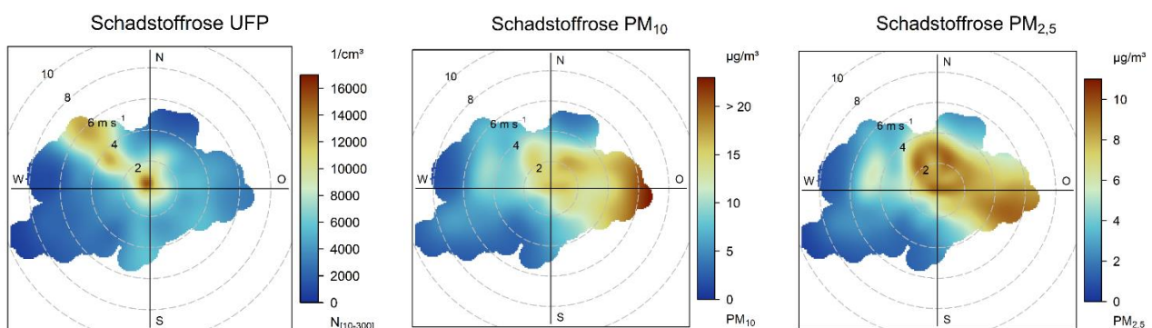
Abbildung 4: Mittlere Konzentrationen von UFP, \text{PM}_{10} und \text{PM}_{2.5} in Abhängigkeit der Windrichtung und der Windgeschwindigkeit an der Messstelle Bernhausen im Jahr 2023
