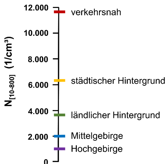
Abbildung 1: Mittlere Partikelanzahlkonzentrationen ( N ) im Größenbereich von 10 nm bis 800 nm für unterschiedliche Stationskategorien in Deutschland gemessen zwischen 2009 und 2014 an GUAN-Messstellen
