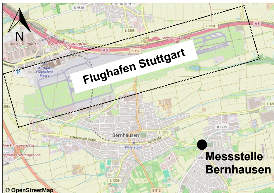
Abbildung 3: Lage der UFP-Messstelle Bernhausen und des Stuttgarter Flughafens
